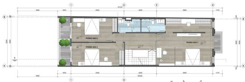
MẶT BẰNG TẦNG 3
