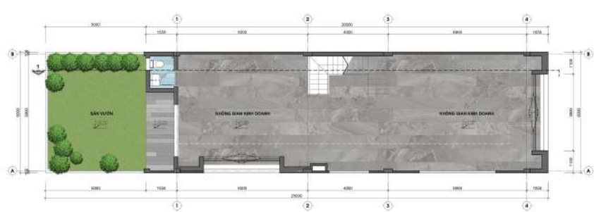
MẶT BẰNG TẦNG 1
