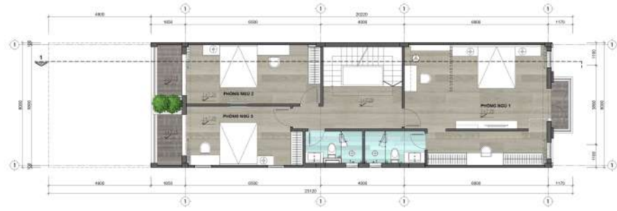
MẶT BẰNG TẦNG 3
