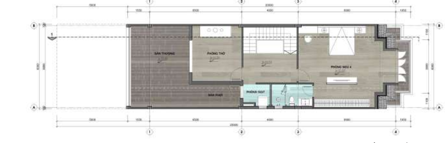
MẶT BẰNG TẦNG 4
