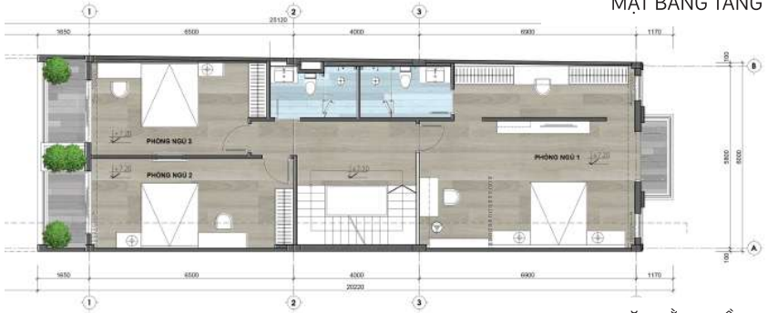
MẶT BẰNG TẦNG 3
