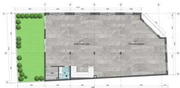
MẶT BẰNG TẦNG 1
