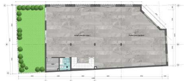
MẶT BẰNG TẦNG 1
